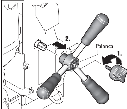
Agarradera de palanca
