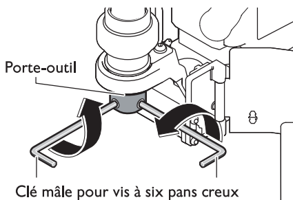
Clé mâle pour vis à six pans creux
