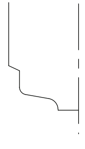
Ogee RCK-496
